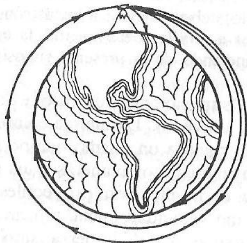
FIGURA 51. — Descripción newtoniana de un proyectil como un satélite. La longitud de la trayectoria crece con la velocidad inicial aplicada al proyectil, de tal modo que cada vez va más lejos alrededor de la superficie curva de la tierra. Cuando la velocidad es suficientemente grande, el proyectil no cae sobre la tierra, sino que continúa moviéndose según una órbita aproximadamente circular.
