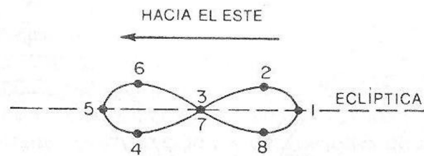
FIGURA 18. — El movimiento en bucle producido por las dos esferas homocéntricas internas. En el sistema completo de cuatro esferas, este movimiento en bucle se combina con el movimiento regular hacia el este de la segunda esfera, movimiento que por sí mismo arrastraría el planeta a lo largo de la eclíptica con velocidad constante. Cuando le añadimos el movimiento en bucle, el movimiento total del planeta adquiere una velocidad variable y abandona periódicamente la eclíptica. Cuando el planeta se traslada sobre el bucle desde 1 a 5, su movimiento total es más rápido que el movimiento medio hacia el este generado por la segunda esfera; cuando retorna desde 5 a 1, su movimiento hacia el este es más lento que el que produce la segunda esfera; cuando está en las proximidades del punto 3, el planeta puede retrogradar hacia el oeste.
