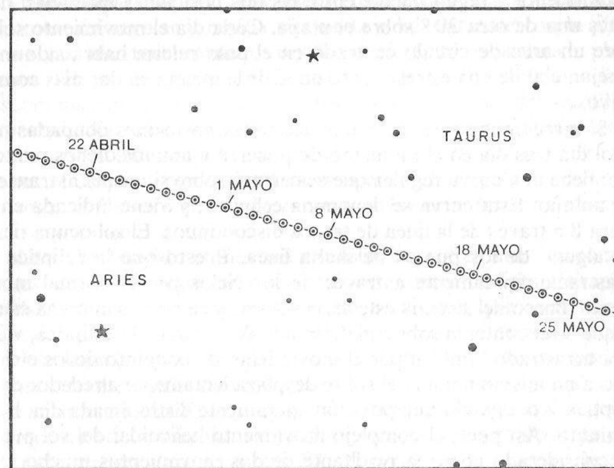
FIGURA 9. — Movimiento del sol a través de las constelaciones Aries y Taurus. Los círculos representan la posición ocupada por el sol en el momento de ponerse durante varias noches sucesivas, de mediados de abril a finales de mayo.
