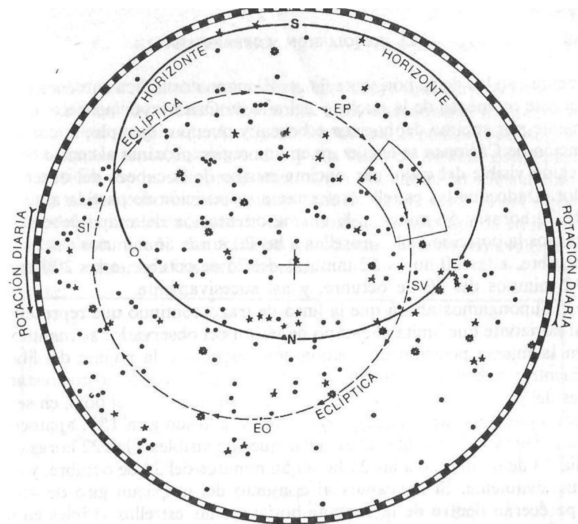
FIGURA 8. — Mapa circumpolar del cielo en el que aparecen las principales estrellas visibles permanentemente para un observador situado alrededor de los 45° de latitud norte. La cruz situada en el centro geométrico del mapa señala la posición del polo celeste.
