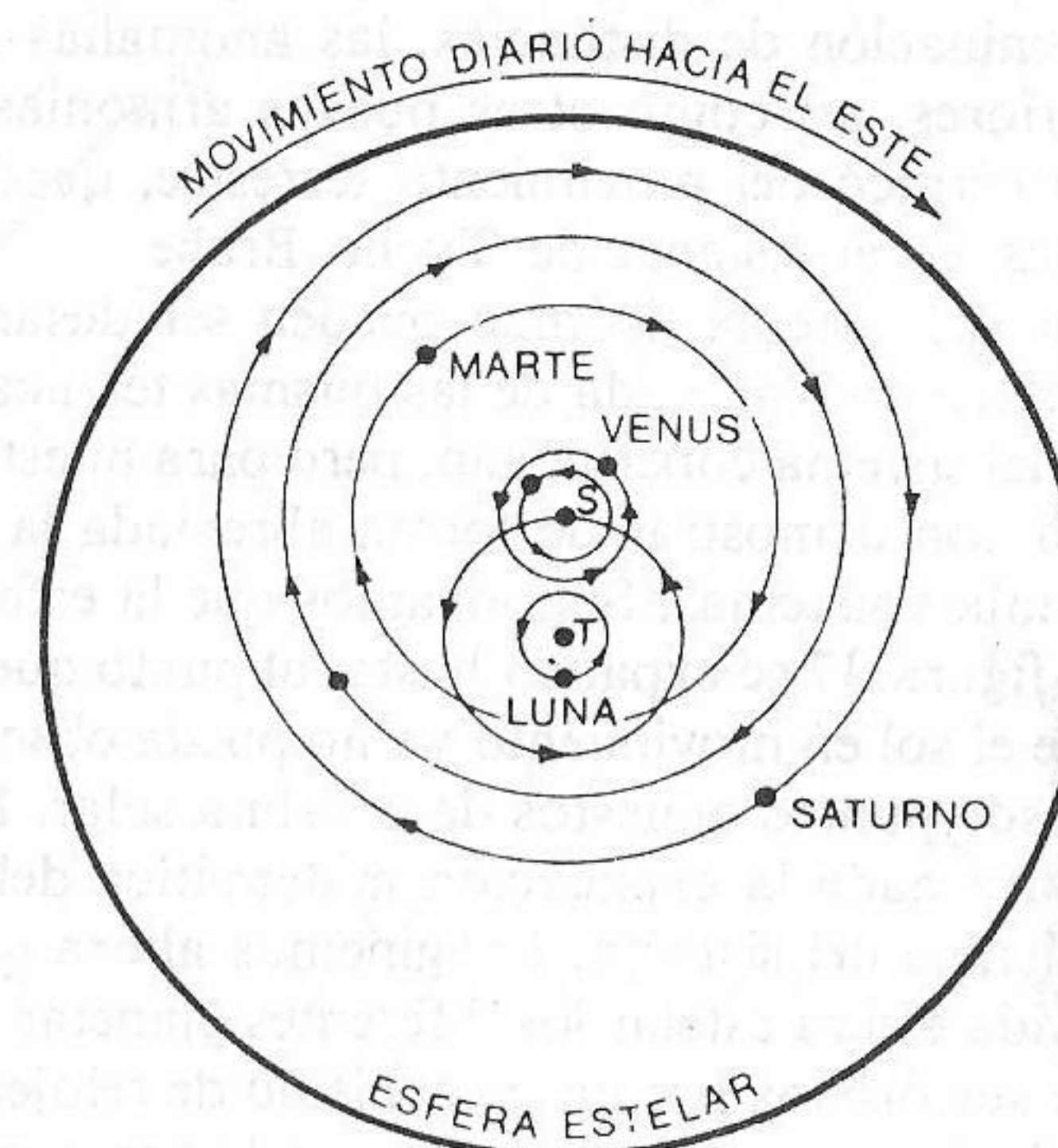
FIGURA 37. — El sistema ticónico. La tierra ocupa una vez más el centro de una esfera estelar en rotación, mientras que la luna y el sol se mueven sobre sus viejas órbitas ptolemaicas. Sin embargo, los otros planetas están situados sobre epí ciclos cuyo centro común es el sol.
