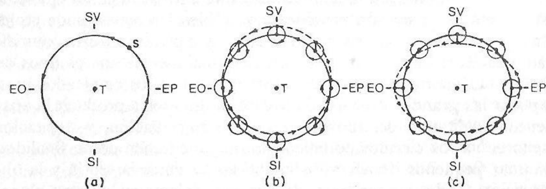
FIGURA 22. — Funciones de un epiciclo menor. En (a) el sol, movido por un solo deferente con centro en la tierra, emplea el mismo tiempo para ir de EO a EP que para retornar de EP a EO . En (b) el movimiento combinado de un deferente y un epiciclo menor arrastra el sol a lo largo de la línea de trazo discontinuo; se necesita, pues, más tiempo para ir de EP a EO que para volver de EO a EP . El diagrama (c) muestra la curva que se genera cuando el epiciclo menor gira con una velocidad doble que la supuesta en la elaboración del esquema (b).
