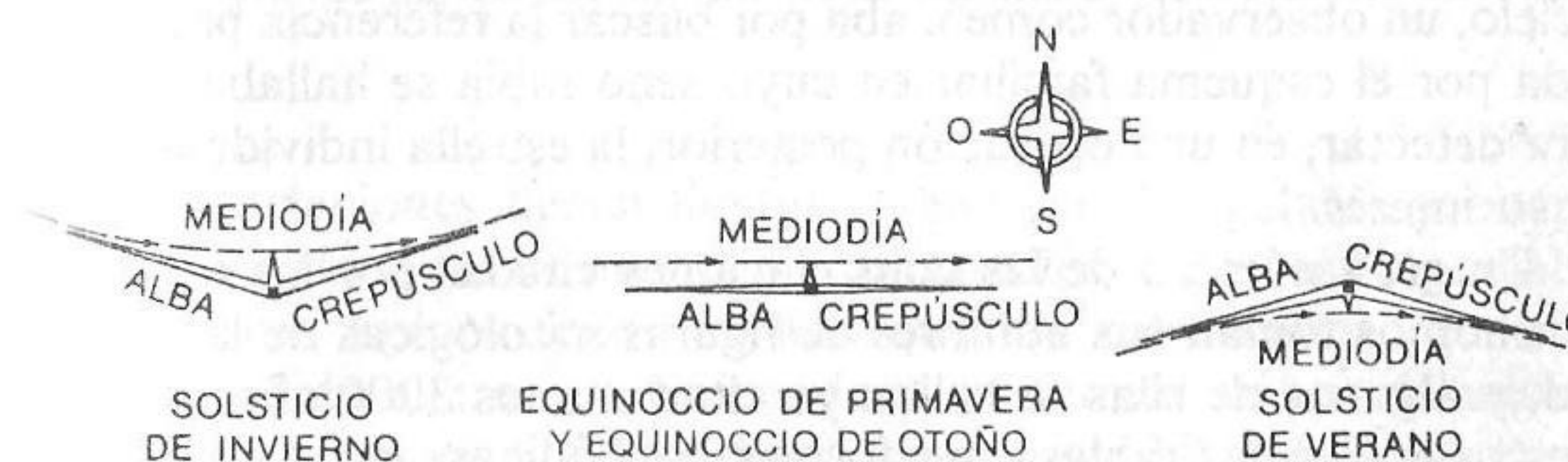
FIGURA 3. — Movimiento de la sombra del gnomon en las zonas tórridas del hemisferio norte durante las diversas estaciones del año.
