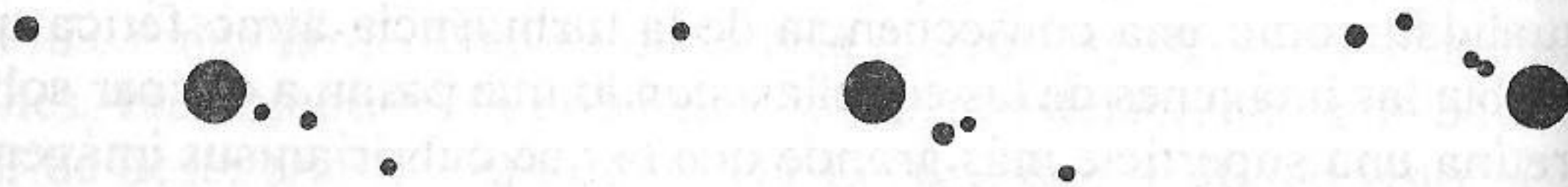
FIGURA 43. — Tres observaciones sucesivas de Júpiter y sus satélites separadas por intervalos de varios días. La disposición constantemente variable de los cuatro pequeños satélites se explica perfectamente suponiendo que están en continua rotación alrededor del planeta.
