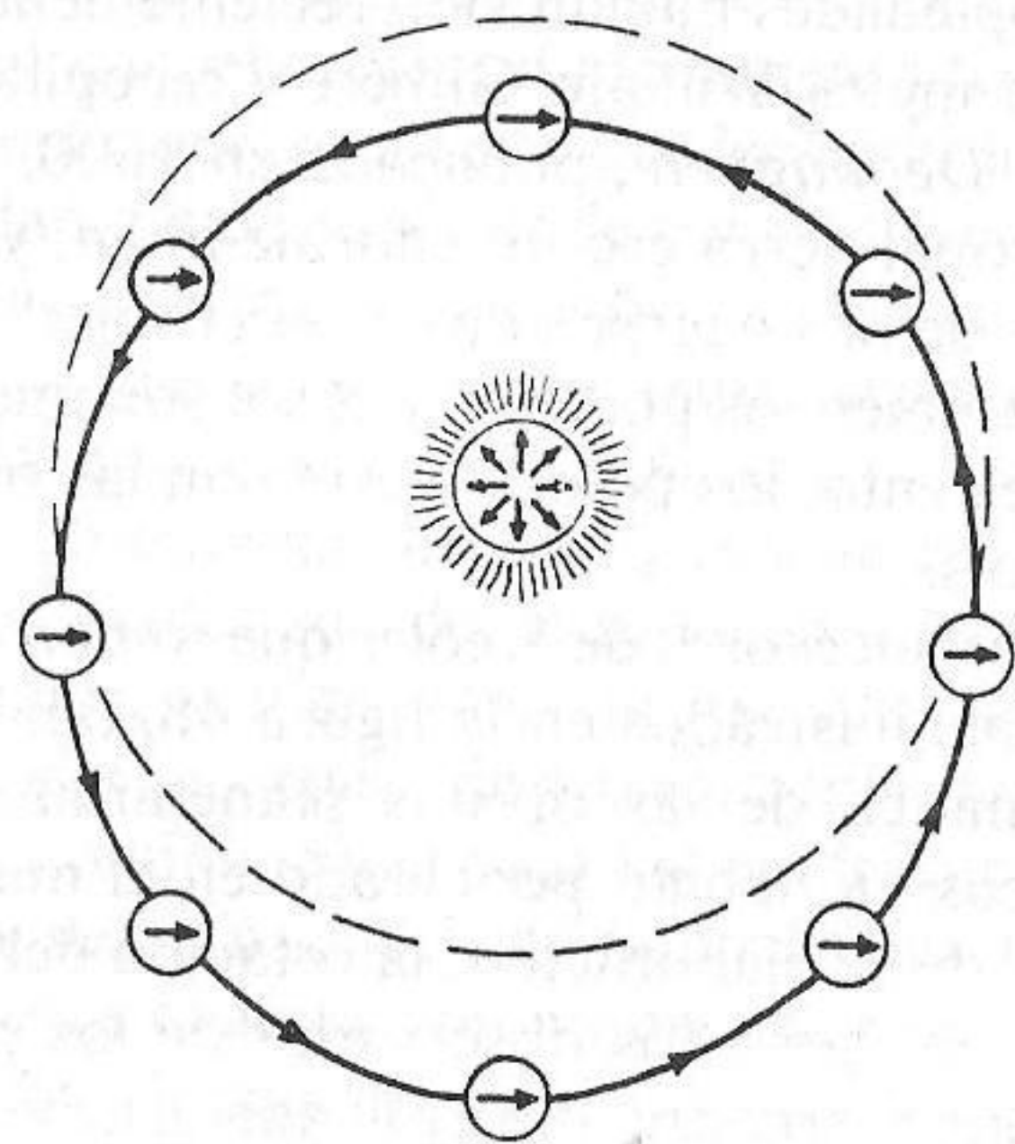
FIGURA 48. — El sistema solar mecánico de Kepler. El sol aparece en el centro del diagrama. De él emanan una serie de rayos, el anima motrix , que, en ausencia de otras fuerzas magnéticas, empujarían al planeta P a lo largo del círculo de trazo discontinuo centrado en el sol. Los imanes que, según Kepler, transforman este movimiento circular en un movimiento elíptico, se hallan representados por pequeñas flechas. El polo sur del sol está en su centro, lugar desde donde no ejerce influencia alguna, mientras que el polo norte se halla uniformemente distribuido por su superficie. El eje magnético de la tierra siempre se mantiene prácticamente paralelo a sí mismo durante el movimiento orbital. Cuando el planeta está a la derecha de una recta vertical imaginaria que pasa por el centro del diagrama, su polo sur está más cercano al sol que su polo norte, por cuya razón se ve atraído hacia el sol de forma progresiva. Durante la otra mitad de su recorrido se invierte la situación y el planeta se ve gradualmente repelido. Dado que la influencia del anima motrix se manifiesta con mayor intensidad en las proximidades del sol, la velocidad orbital del planeta siempre será inversamente proporcional a su distancia al mismo.
