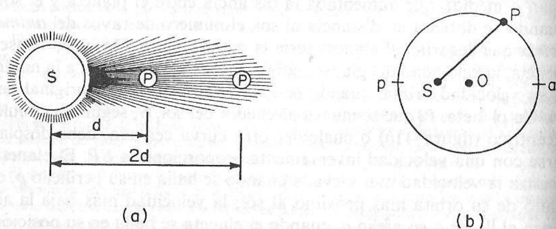
FIGURA 41. — La primitiva ley de velocidades enunciada por Kepler. El diagrama (a) muestra los rayos del anima motrix que emanan del sol, ilustrando la teoría física de la cual Kepler dedujo su ley. El diagrama (b) muestra en qué forma puede ser aplicada esta ley a un planeta que se mueva sobre una excéntrica.
