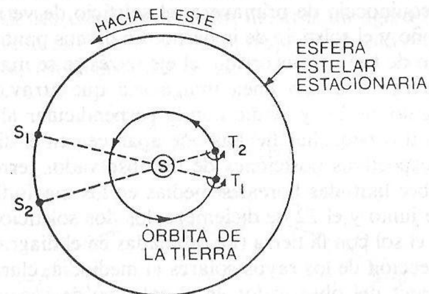
FIGURA 28. — Cuando la tierra se desplaza de T_1 a T_2 a lo largo de su órbita copernicana, la posición aparente del sol sobre la esfera de las estrellas pasa de S_1 a S_2 .
