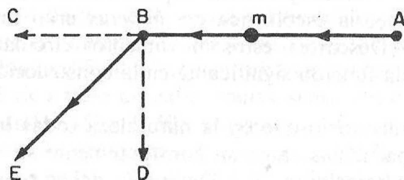
FIGURA 46. — Efecto de un impulso sobre un movimiento inercial. En el punto A , el cuerpo m recibe un violento impulso que lo lanza hacia B . Si no actúa ninguna fuerza adicional el cuerpo se trasladará de A a B a lo largo de una línea recta y con una velocidad constante. Si cuando llega a B recibe un segundo impulso en la misma dirección, continuará su movimiento en línea recta hacia C , pero aumentará su velocidad de traslación. Si se le aplica una fuerza en sentido opuesto, puede continuar su camino hacia C con menor velocidad que la que poseía al llegar a B o bien, en el caso de que la nueva fuerza aplicada sea suficientemente grande, podrá retroceder hacia A . Finalmente, si cuando llega a B el cuerpo recibe un impulso lateral hacia D , iniciará un nuevo movimiento inercial a lo largo de la línea oblicua BE . Puede considerarse que el movimiento inercial a lo largo de BE es la resultante de dos movimientos inerciales simultáneos, uno según la dirección BC , producido por la primera fuerza aplicada en A , y otro según la dirección BD , producido por el segundo impulso lateral recibido al llegar a B .
