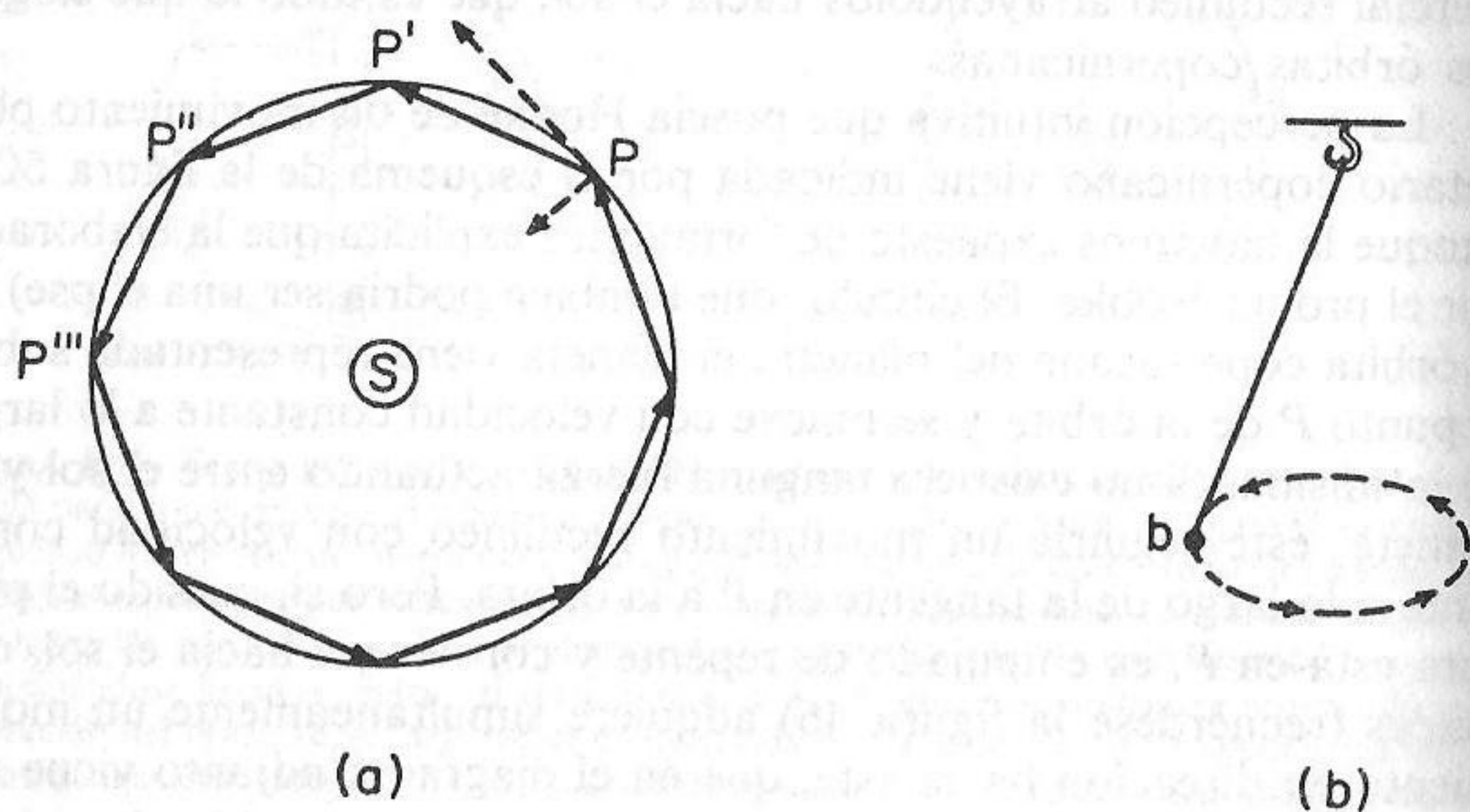
FIGURA 50. — Teoría planetaria de Hooke (a) y su demostración por medio del péndulo cónico (b). En el diagrama (a) el planeta se ve sometido en cada uno de los puntos P, P', P'', \dots a un impulso instantáneo que lo dirige hacia el sol S . A cada nuevo impulso queda modificada la dirección del movimiento inercial del planeta, y el resultado de la acción de todos ellos es un movimiento a lo largo del perímetro de un polígono. Incrementando el número de puntos en los que el planeta es empujado hacia el centro, crece el número de lados del polígono. En el límite, la acción permanente de una fuerza atractiva central produce una órbita circular. La circularidad de este movimiento puede demostrarse físicamente mediante el aparato representado en el diagrama (b). Si sólo recibe un impulso lateral, el plomo b del péndulo se verá atraído a causa de su propio peso hacia un punto próximo al centro del círculo de trazo discontinuo. Sin embargo, si lo que se comunica al plomo es un impulso en una dirección perpendicular al hilo del que se halla suspendido, su peso le llevará forzosamente a moverse según una curva. Si la intensidad del impulso es la adecuada, el movimiento del plomo tendrá lugar a lo largo de un círculo horizontal o de una órbita alargada muy similar a una elipse.
