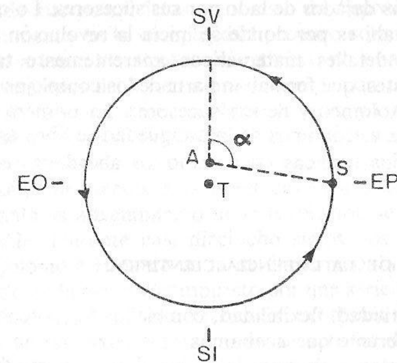
FIGURA 25. — El ecuante. El sol S se desplaza a lo largo de un círculo centrado en la tierra, pero lo hace con velocidad variable determinada por la condición de que el ángulo \alpha gire uniformemente en función del tiempo.
