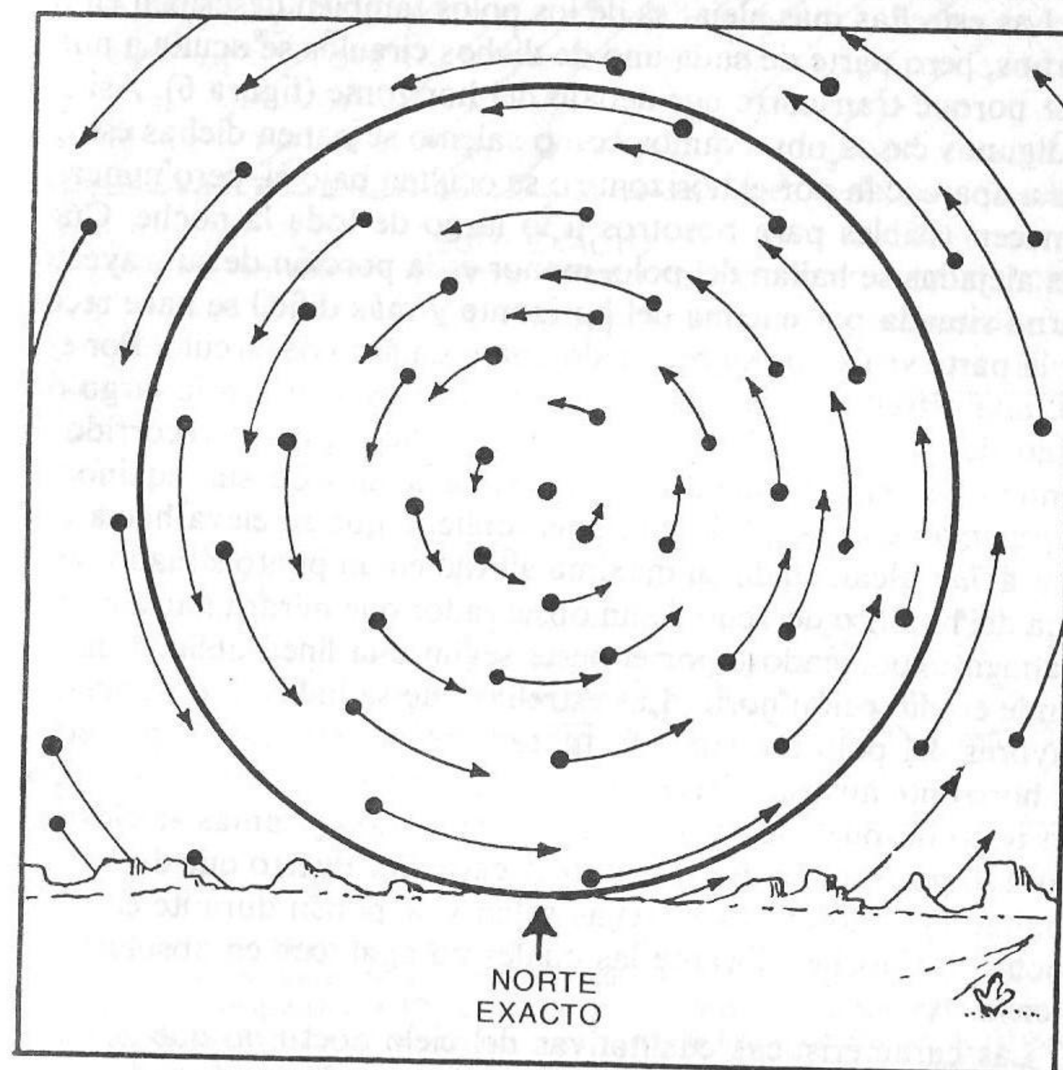
FIGURA 6. — Conjunto de arcos de círculo descritos por algunas estrellas del hemisferio norte durante un periodo de dos horas. La circunferencia de trazo grueso tangente al horizonte separa las estrellas circumpolares de las que salen y se ponen.
