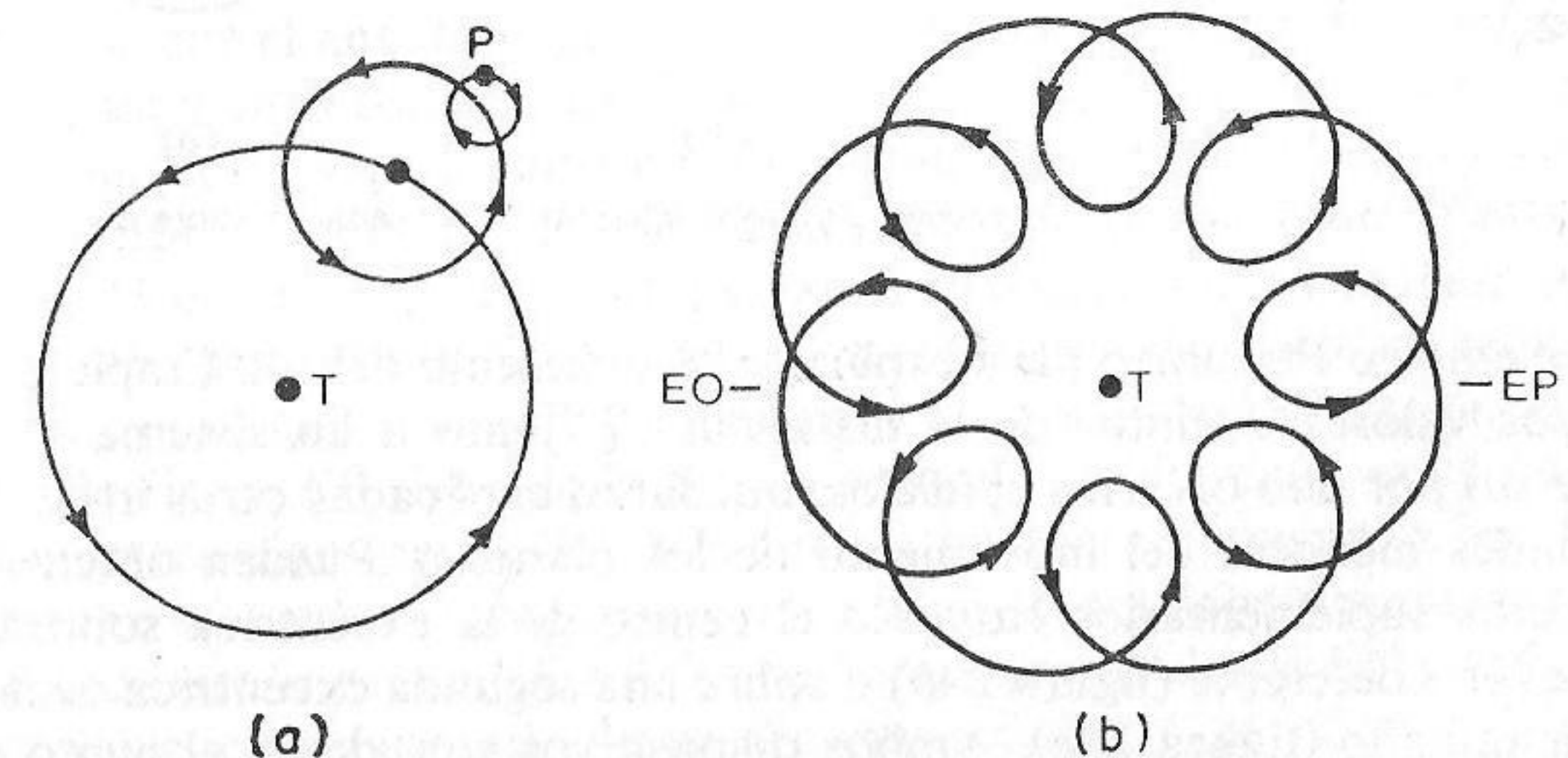
FIGURA 23. — (a) Un epiciclo, sobre un epiciclo, sobre un deferente; (b) camino típico engendrado en el espacio por tal sistema compuesto de círculos. Para simplificar, se ha representado una curva que se cierra sobre sí misma, situación que no se produce en el movimiento real de los planetas.
