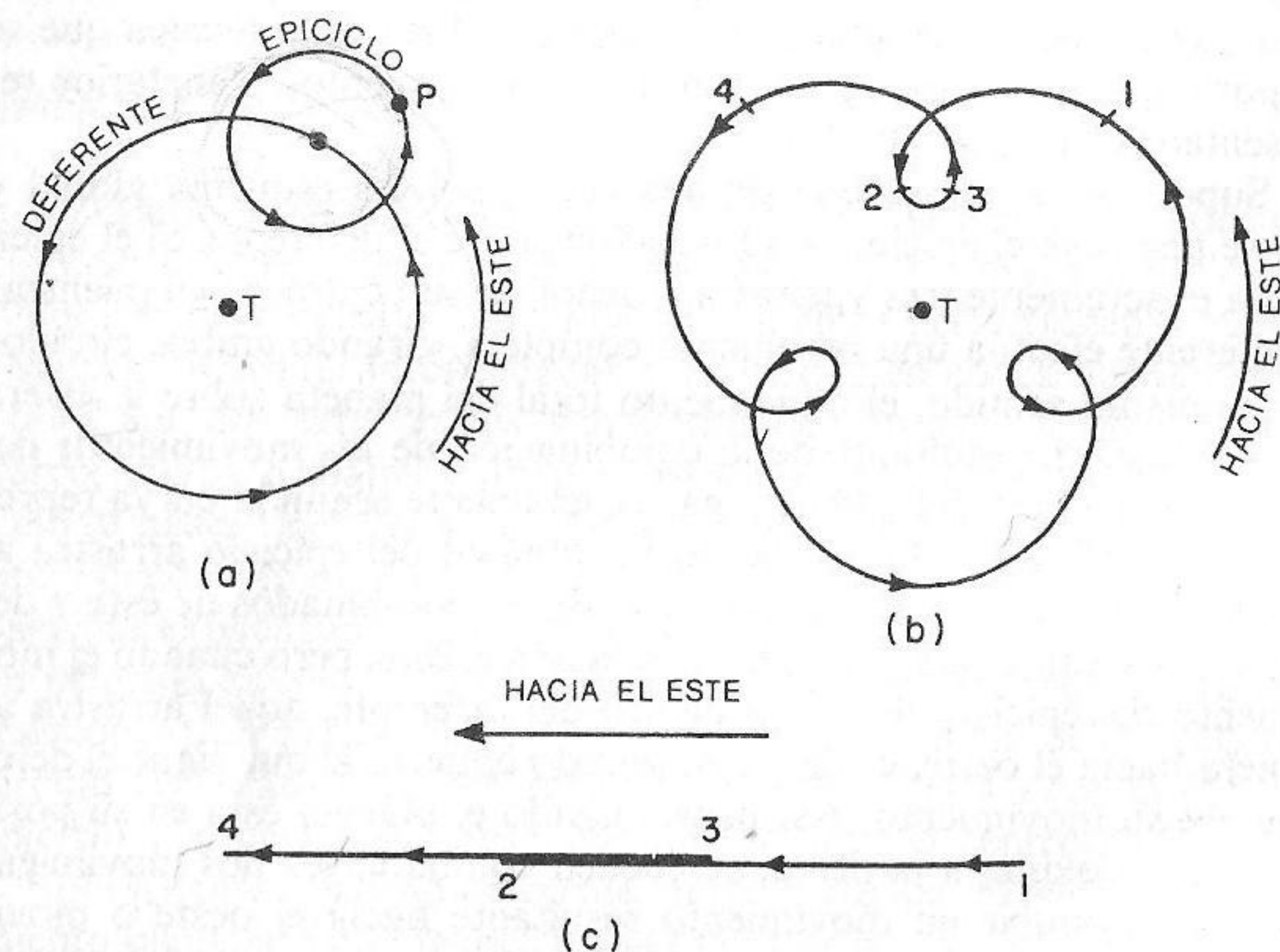
FIGURA 19. — El sistema básico epiciclo-deferente. En (a) se representa un caso típico de epiciclo y deferente; en (b) aparece el movimiento en bucle generado por tal sistema en el plano de la eclíptica; en (c), se ofrece parte del movimiento representado en (b), el trayecto 1-2-3-4 tal como es visto por un observador situado sobre la tierra central T.
