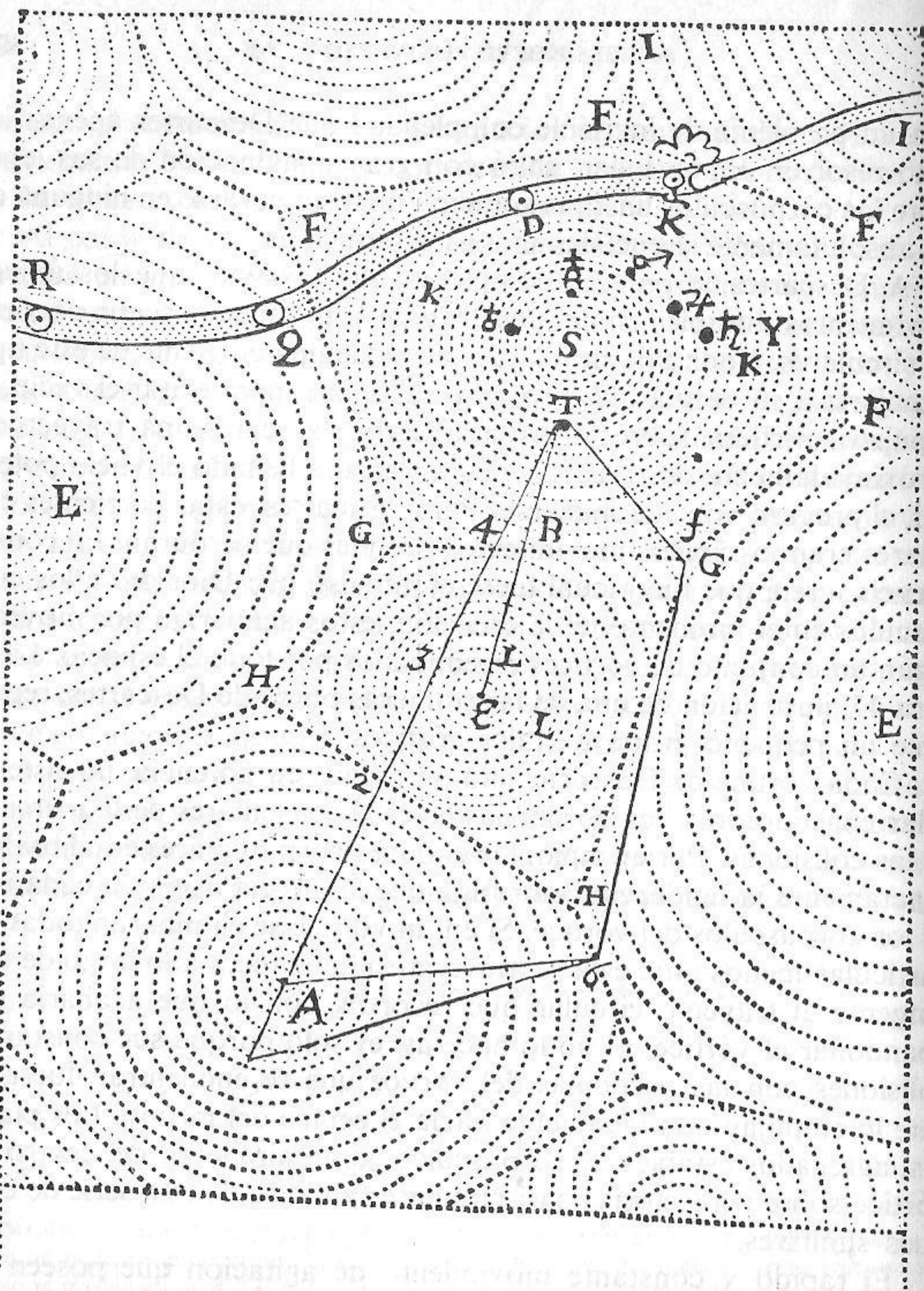
FIGURA 47. — La cosmología de los torbellinos de Descartes, reproducida de su obra Le monde ou le traité de la lumière . Los puntos S , E , A y ε son los centros de los torbellinos. Los rápidos movimientos en torbellino de los corpúsculos centrales los convierten en luminosos, por lo que actúan a modo de estrellas. Los diversos círculos punteados, que no es necesario que conformen circunferencias perfectas, representan los caminos descritos por las corrientes corpusculares, eternamente en rotación, que constituyen el torbellino. Los puntos negros situados alrededor del centro S del torbellino son los planetas, que se ven arrastrados a lo largo de sus respectivas órbitas por el movimiento de los torbellinos. El cuerpo C , situado en la parte superior del diagrama, es un cometa que atraviesa los diferentes torbellinos en una región en la que su movimiento es demasiado lento para constreñirlo sobre una órbita circular continua. El espacio exterior al diagrama está asimismo lleno de torbellinos y cada uno de ellos, al menos potencialmente, representa la localización de un sistema solar en el seno del universo copernicano de Descartes poblado por una infinidad de mundos.
